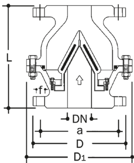
DN 50-125
