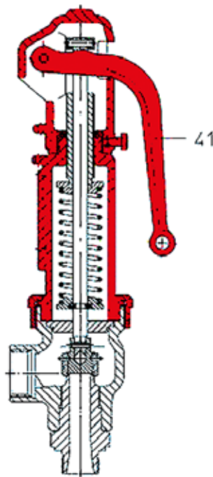
Figur 942 öppet lättverk sluten huv
