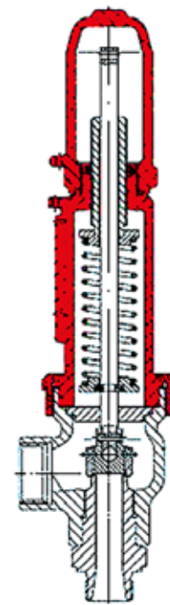
Figur 943 gastät kåpa sluten huv
