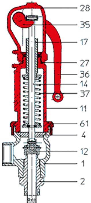
Figur 941 slutet lättverk sluten huv
