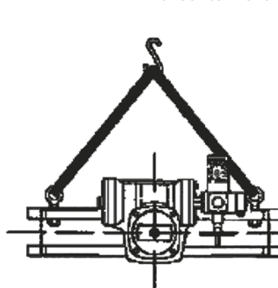
Horisontell ventil
